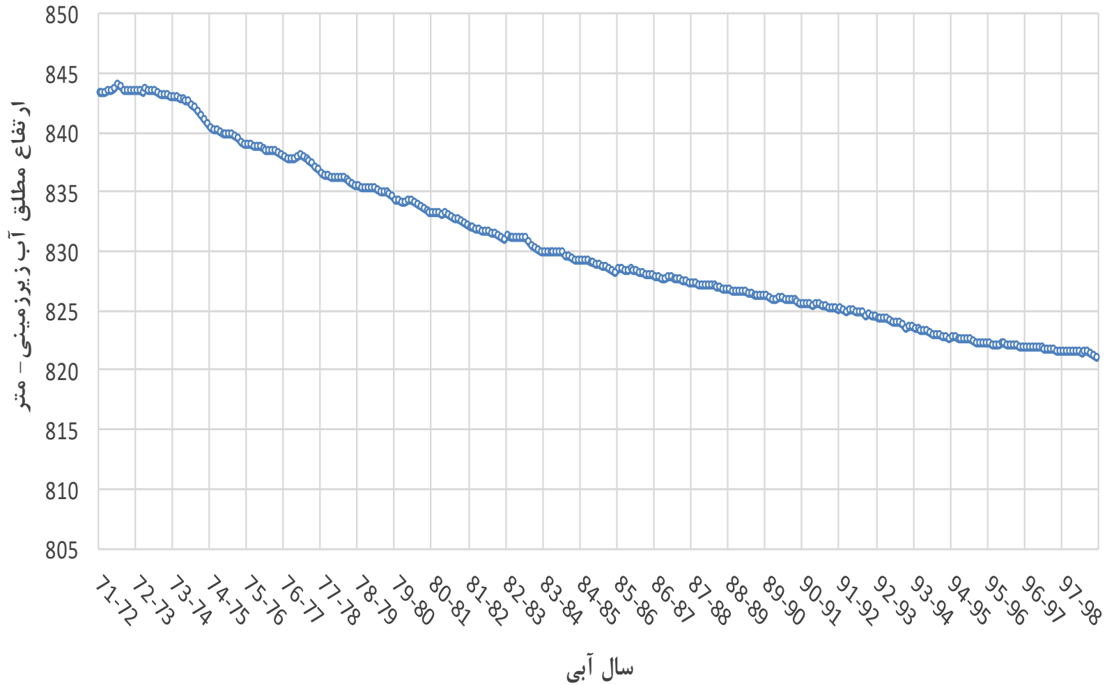
هیدروگراف واحد آبخوان جنگل
