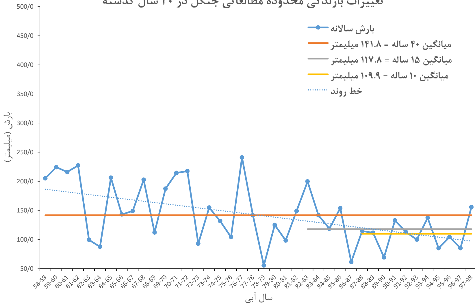
تغییرات بارندگی محدوده مطالعاتی جنگل در ۴۰ سال گذشته
