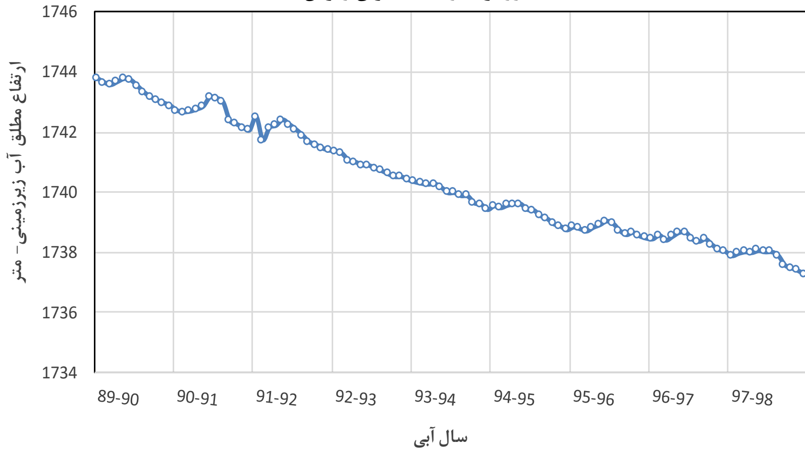
هیدروگراف واحد آبخوان ریوش
