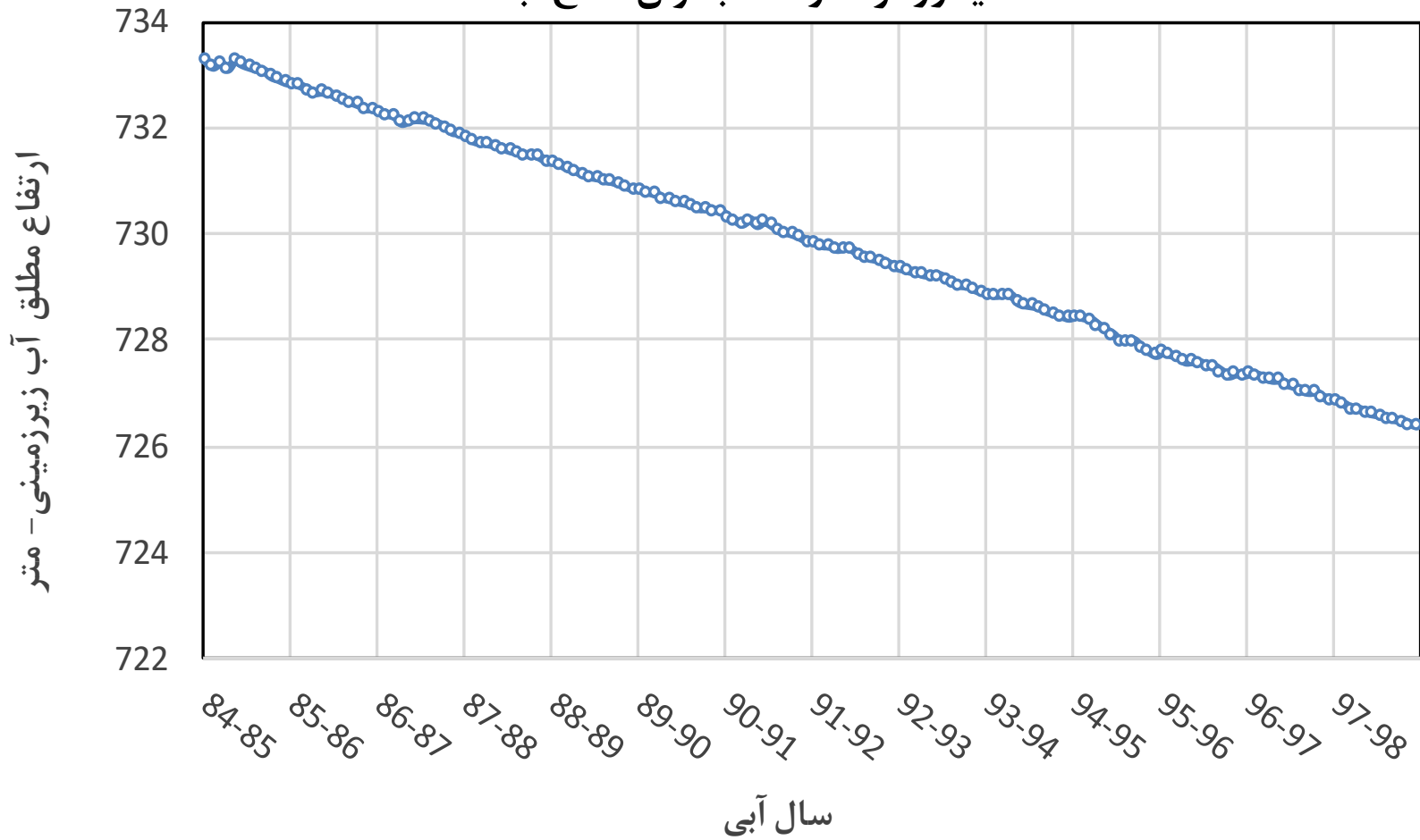
هیدروگراف واحد آبخوان صالح آباد
