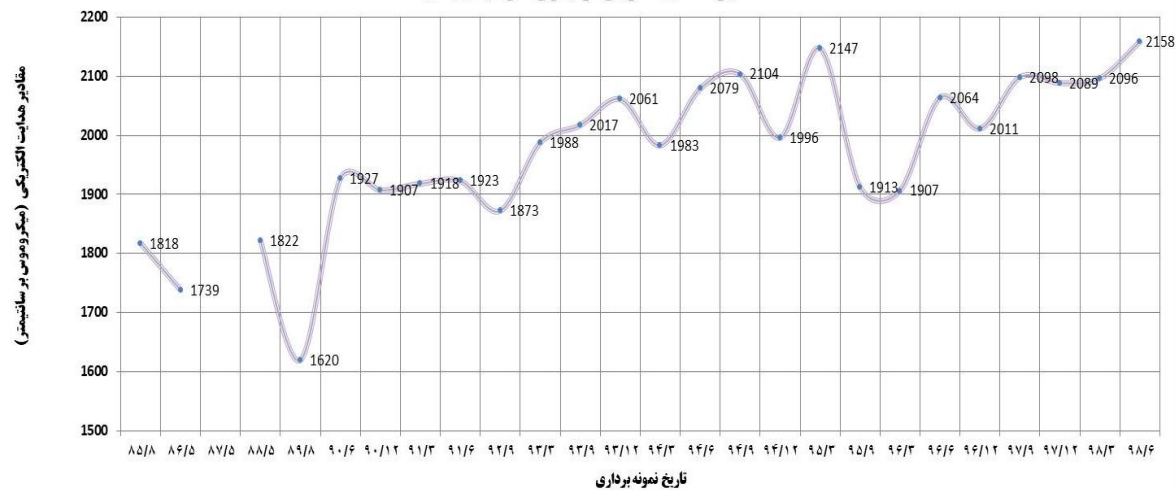
تغییرات هدایت الکتریکی در آبخوان صالح آباد ۸۵ تا ۹۸
